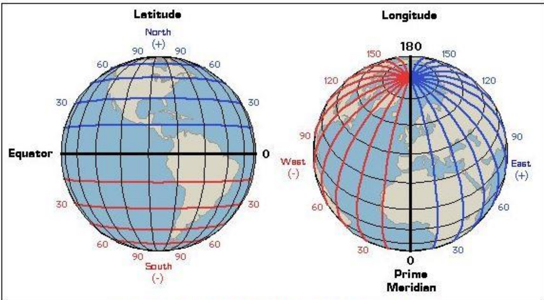
Earth Latitude and Longitude in Degrees (3 6 9)
